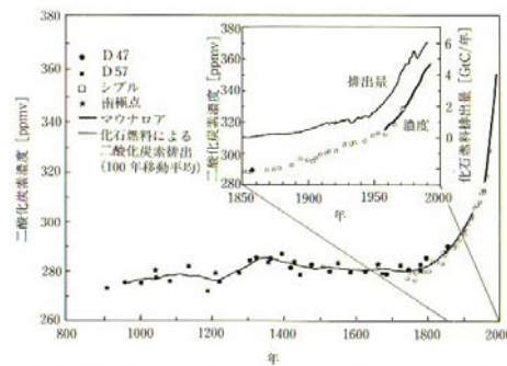
図 5-1 過去 1000 年間の氷床に残された二酸化炭素の大気中濃度の記録 (気象庁編、「地球温暖化監視レポート'94」)
