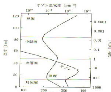
図 2-3 大気の大気圧、温度、オゾン濃度の高度分布
